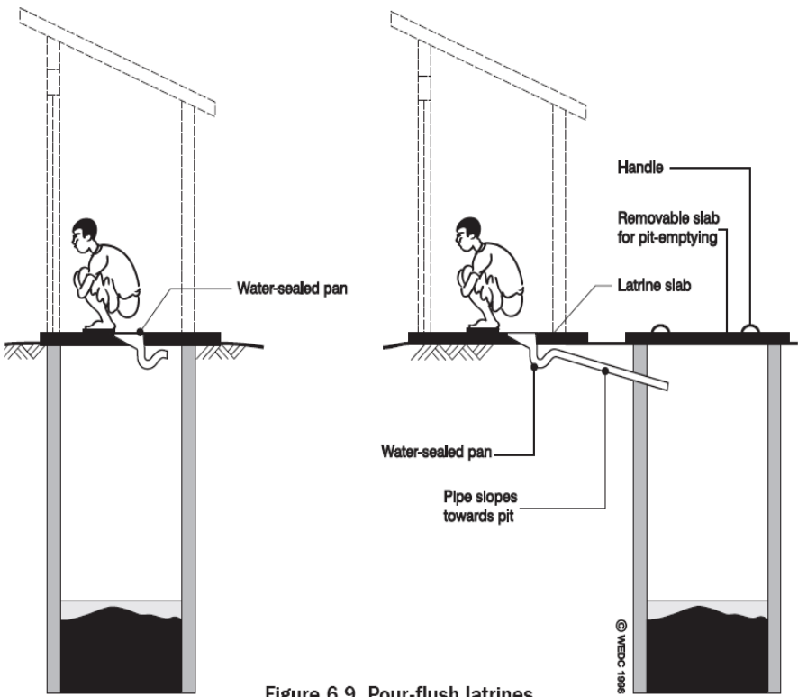
Figure 6.9. Pour-flush latrines
